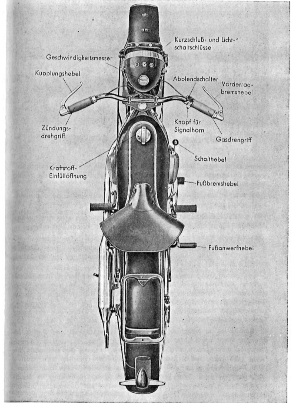
Abb. 6 Die Bedienungshebel der R 3- und R 4-Maschine
