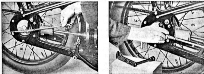
Abb. 11. Nachstellen der Hinterradbremse bei der R 2-Maschine
