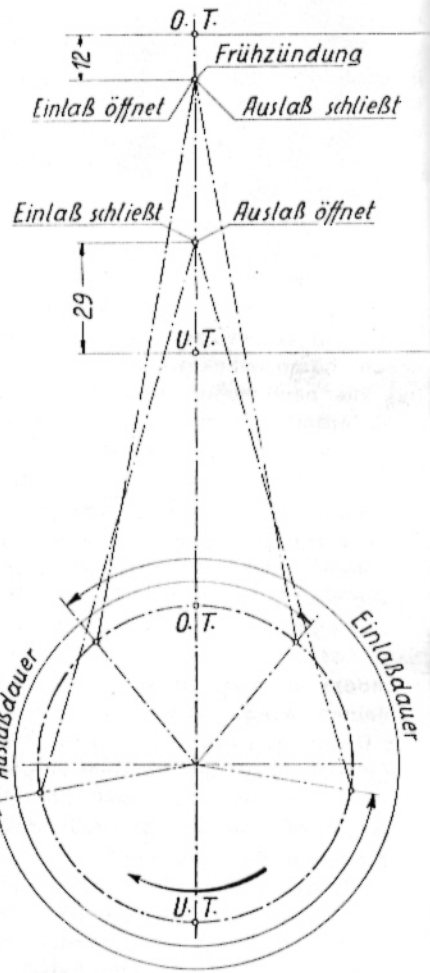
Abb. 34. Einstellschaubild der R 3- u. R 4-Maschine
