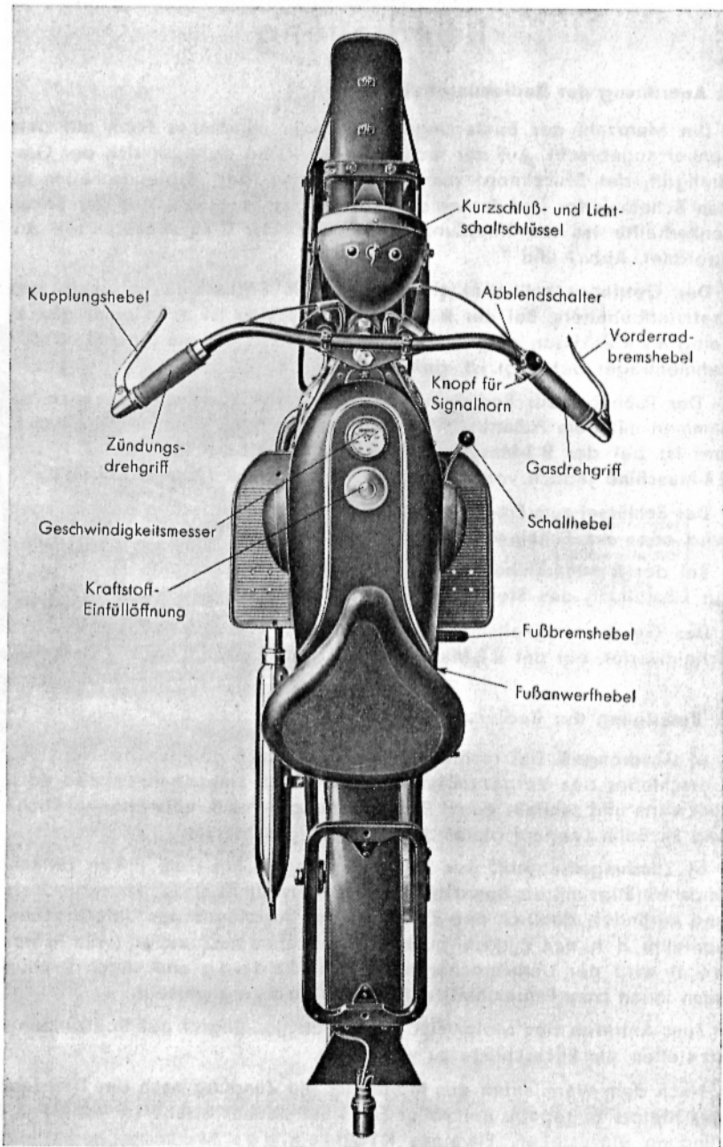
Abb. 5 Die Bedienungshebel der R 2-Maschine
