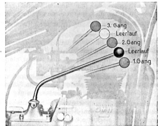
Abb. 10 Schalthebelstellungen bei der R 2-Maschine
