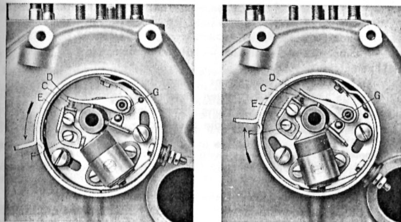
Abb. 13. Unterbrecherkontakte
