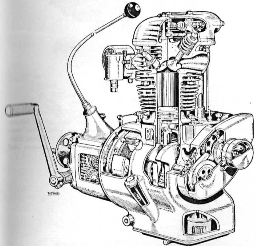
Abb. 17. Motor-Getriebeblock der R 4-Maschine
