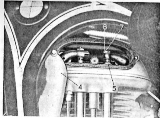
Abb. 16. Kipphebel der R 4-Maschine
