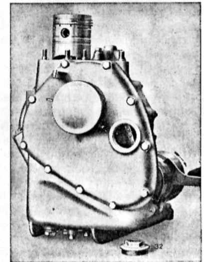
Abb. 35. Nachspannen der Pleuelstößelrad bei der R 2-Maschine
