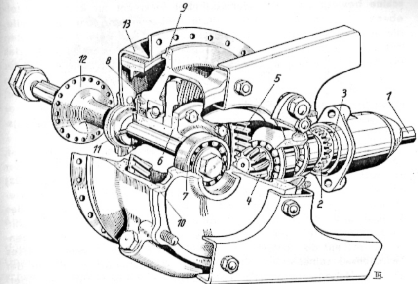
Abb. 29. Kraftübertragung im Kardangehäuse
